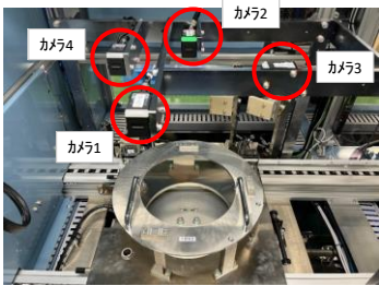
マスタチェック治具
